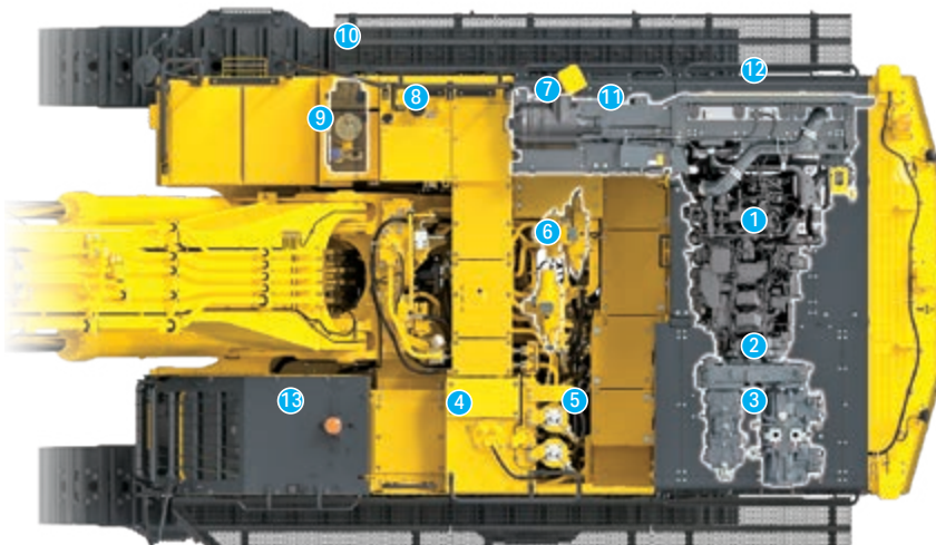
Breiter Trittsteg in der Mitte für Wartungsarbeiten
